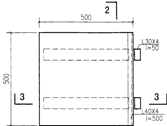
走道板 DB-1a
