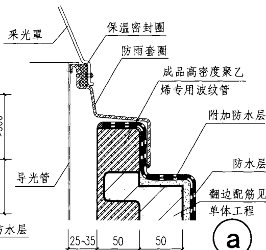
导光管采光系统构造节点
