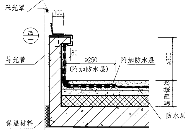
① 卷材、涂膜屋面 (有保温层)
