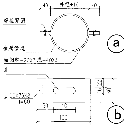
② 管径 300 ~ 1000
