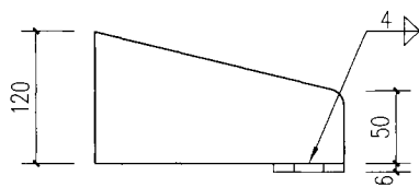
支架钢板
