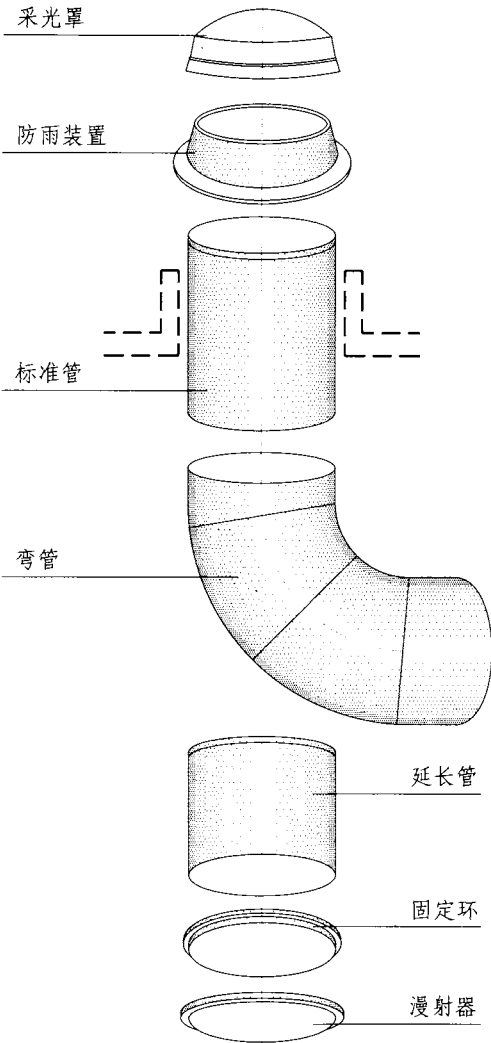
导光管采光系统结构构成示意图
