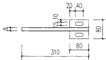
支架钢板
