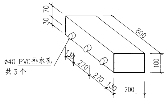
(b) 预制混凝土堵头
