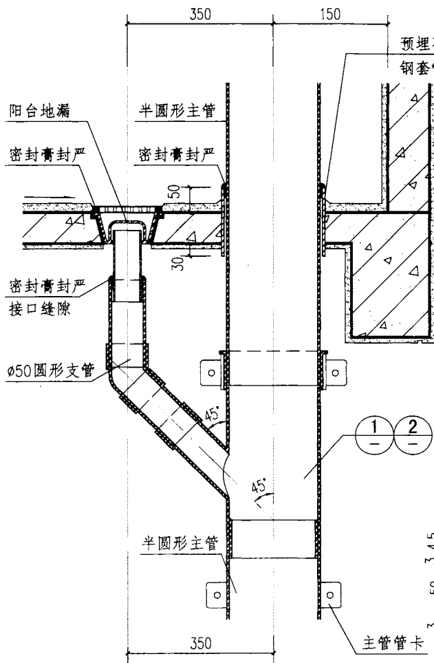
阳台有组织排水剖面示意图
